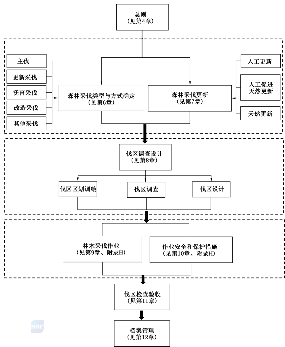
图 1 林木采伐程序流程图
