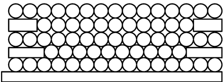
图 H.6 实楞
